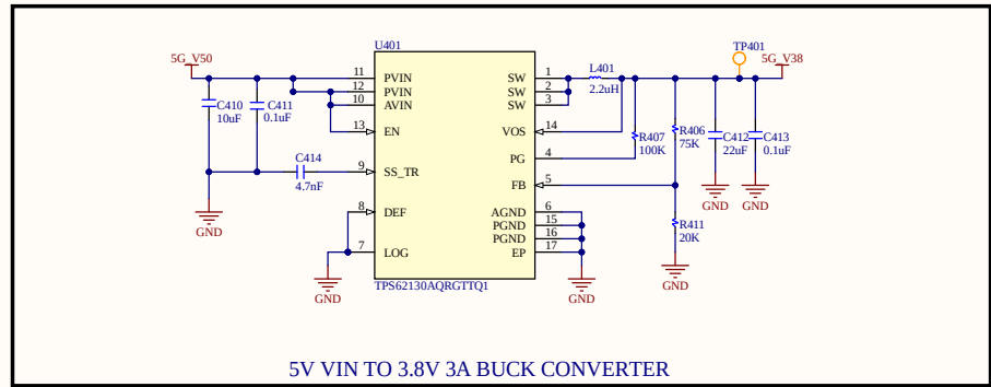
5V VIN TO 3.8V 3A BUCK CONVERTER
